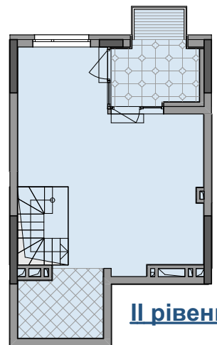
План квартири без перегородок
