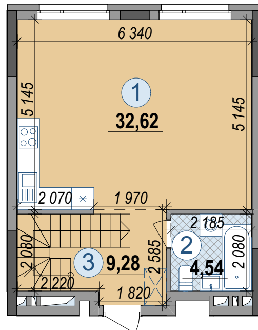
I рівень
