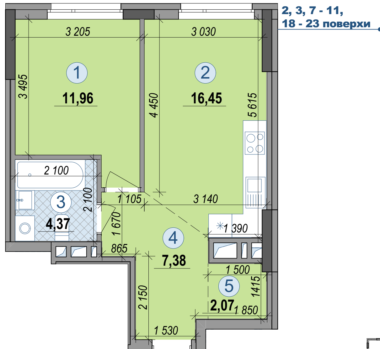
План поверху
