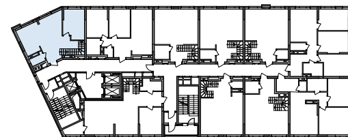
План 25 поверху
